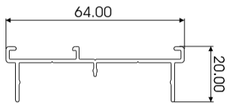
ROUGE FRAME JAMB W34247
