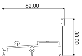
ROUGE FRAME SILL W34200
